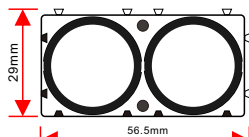
电池支架
